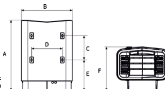
Dimensions des poêles (cf tableau ci-dessus)
